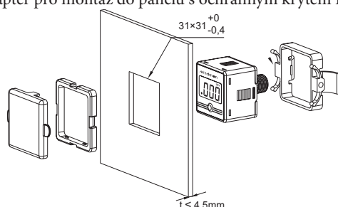
Adaptér pro montáž do panelu s ochranným krytem PA-D
